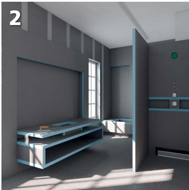
2 Conçu avec les panneaux wedi, isolant et prêt à carrelé
